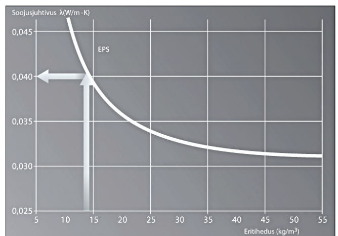
Soojusjuhtivuse sõltuvus valge EPS-i tihedusest
